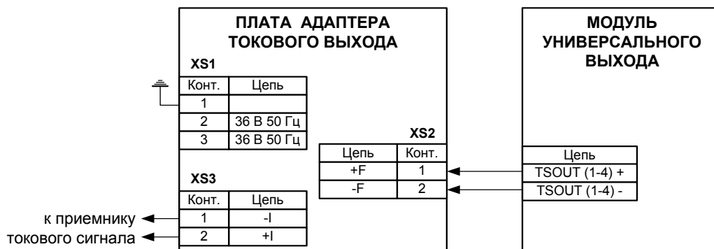
Рис.Г.2. Схема подключения платы адаптера.
