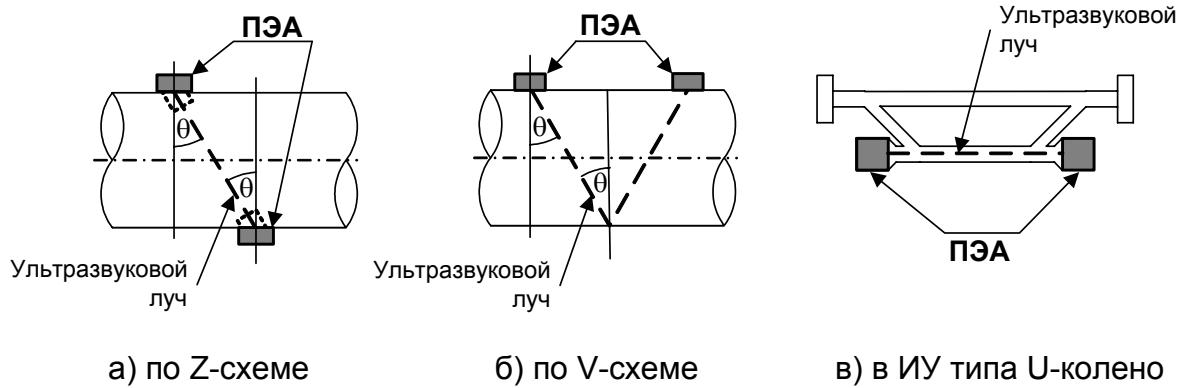
Рис. 2. Схемы установки ПЭА на трубопроводе.
